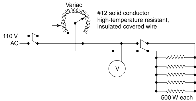
FIGURE 6-10.4.2(d) Radiant test apparatus.
