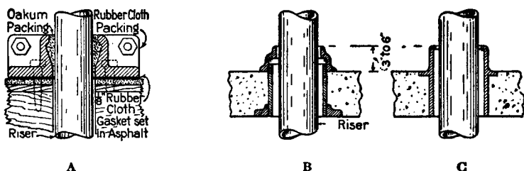
Fig. 4312. Watertight Riser Sleeves.
