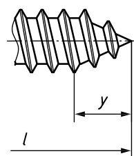
c) Type C (cone end)
