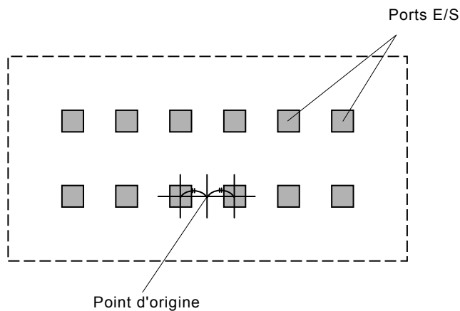
Figure 9 – Définition du point d'origine 2): détermination d'un point d'origine à un endroit où il n'y a pas de port (un point milieu de deux ports adjacents au centre de la ligne du bas est utilisé comme origine)
