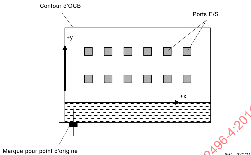
Figure 14 – Point d'origine et direction de l'axe de coordonnées (combinaison des Figures 12 et 13)
