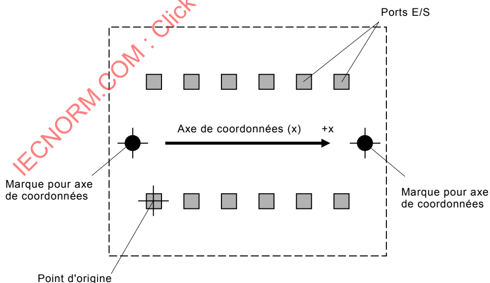
Figure 15 – Utilisation du système de coordonnées interne et du système de coordonnées externe: interne pour le point d'origine (port d'entrée/sortie optique spécifique) et externe pour la direction de l'axe (structure dédiée)
