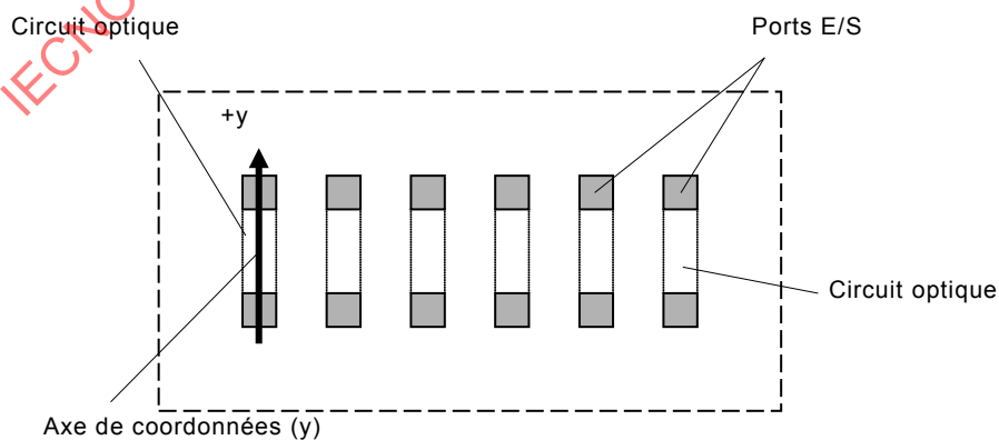
Figure 11 – Définition de la direction de l'axe des coordonnées 2): suivant un circuit optique spécifique (uniquement si le fil est reconnaissable)
