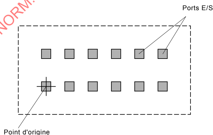
Figure 8 – Définition du point d'origine 1): un port spécifique est utilisé comme point d'origine
