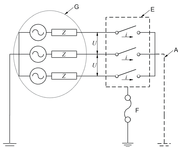
Figure 2b – Circuit d'essai avec point de court-circuit
