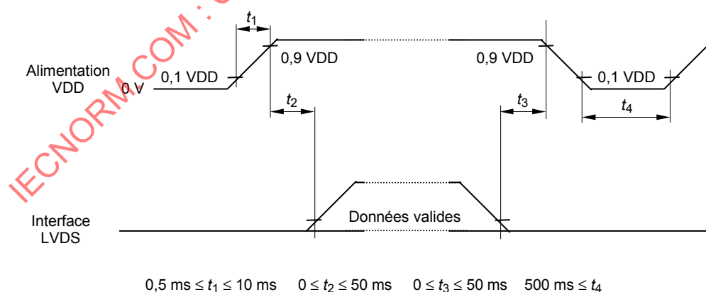
Figure A.3 – Diagramme de séquençement logique des signaux de puissance et LVDS
