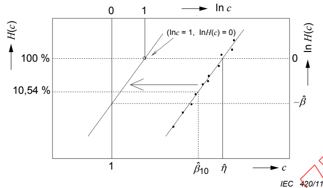
Figure A.4 – Estimation des paramètres de distribution
