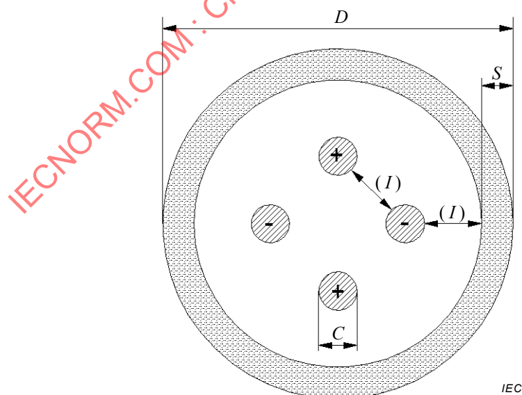
Figure 2 – Section transversale du câble et du couple thermoélectriques duplex
