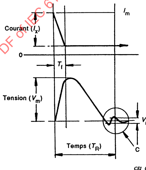
Figure 2 – Débranchement d'une charge résistive aux bornes de sortie
