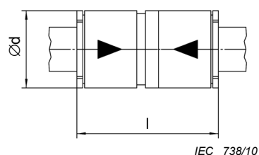
Figure 6b – Variante de boîtier 2
