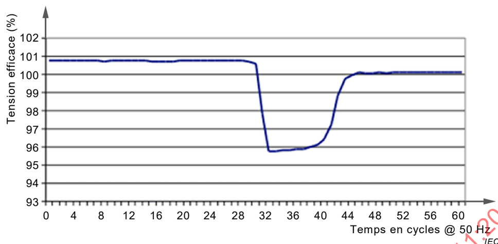
Figure A.1 – Diagramme type de variation de la tension efficace au démarrage du moteur
