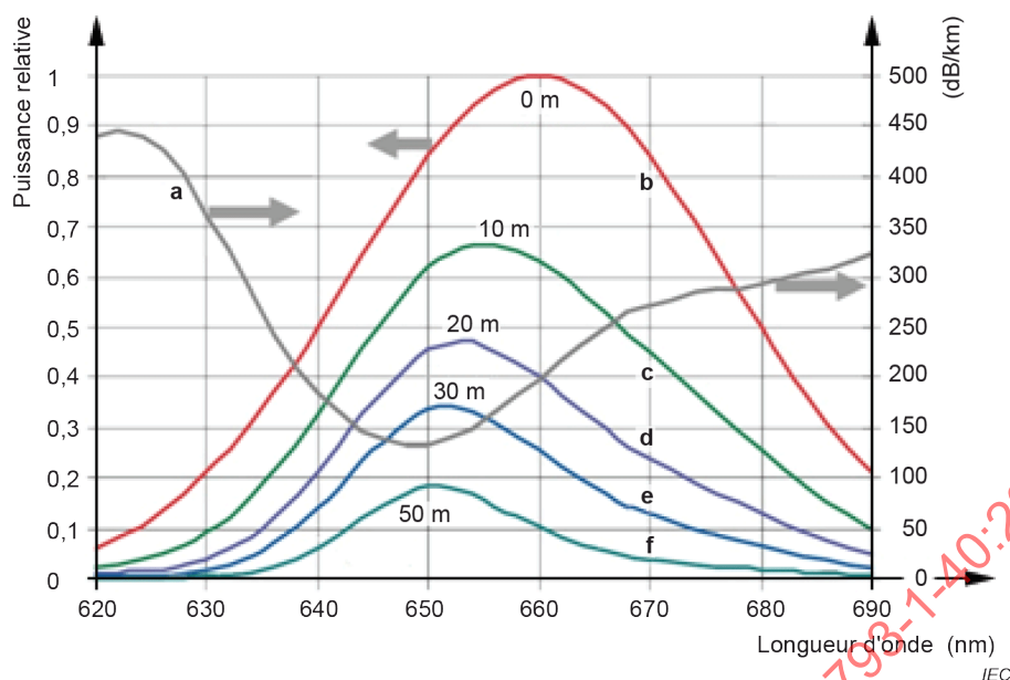
Figure A.9 – Une source de large spectre (ligne "b") peut provoquer des erreurs de mesurage de l'affaiblissement en raison des variations brusques de l'affaiblissement spectral de fibres à cœur polymère (ligne "a")
