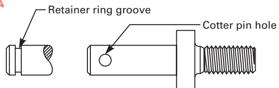
Collar Stud
